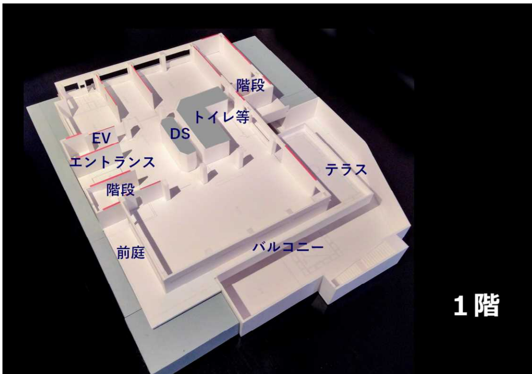
1階スケルトン模型 ※構造上主要な柱、壁だけを残した骨組模型
